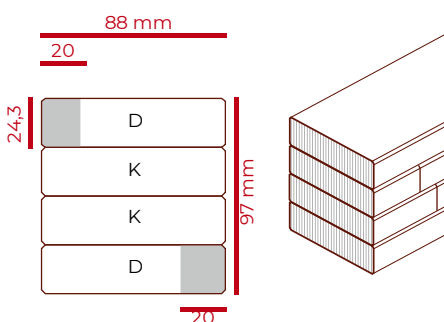
BEISPIEL KANTEL 97 x 88 mm »DKKD«
