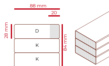
BEISPIEL KANTEL 84 x 88 mm »DKK«
