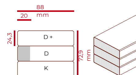
BEISPIEL KANTEL 73 x 88 mm »D+DK«
